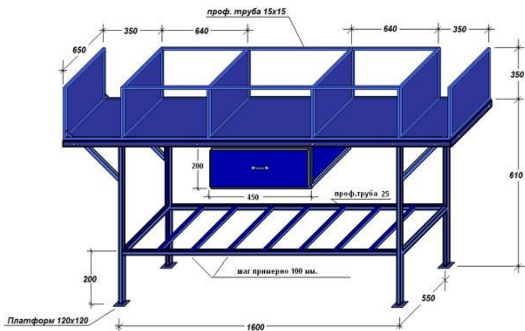
Стол фасовщика СФ-2
