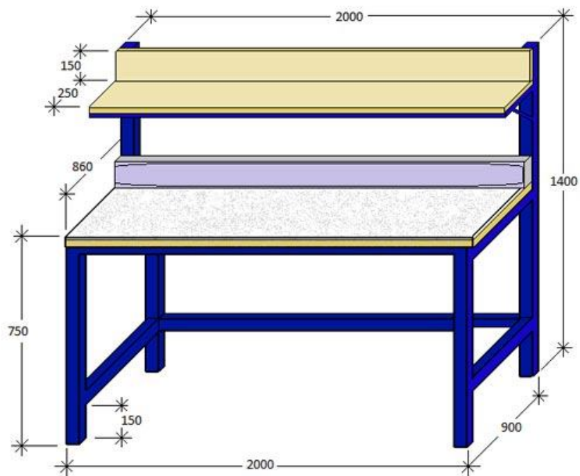
Стол фасовщика СФ-2
